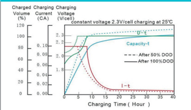
Характеристики заряда
