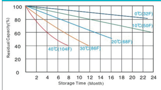
Характеристики хранения
